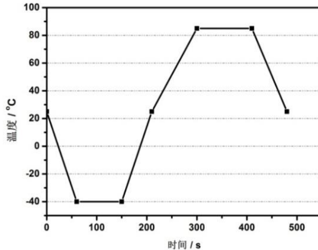
图 5.1 温度循环中温度时间曲线
